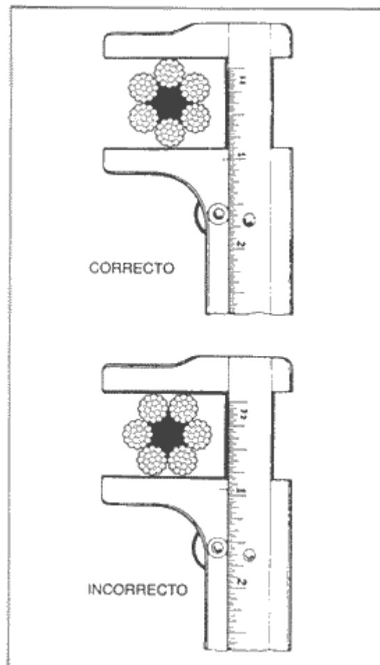
Verdadero diámetro
